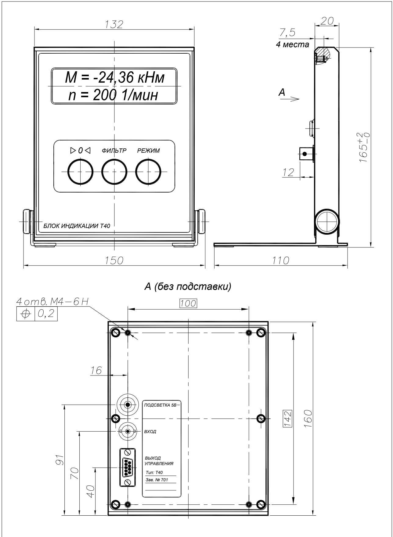
Рис. 1. Габаритные и установочные размеры
